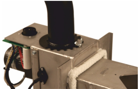
hořák
